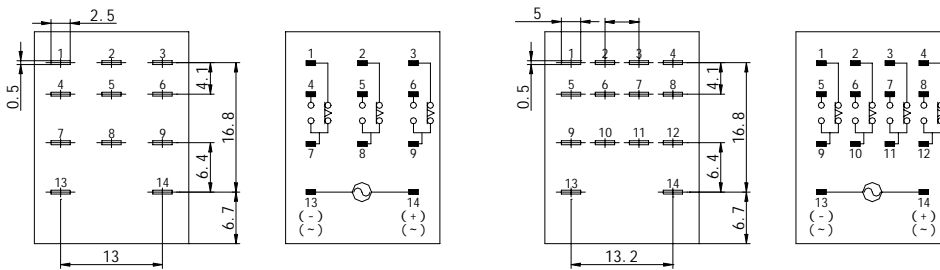
3Z接线图
